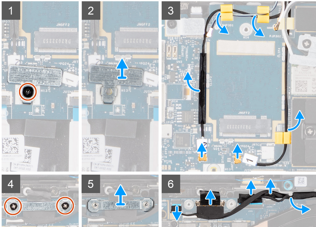
Figure 3. Assemblage d'écran avec antenne WLAN et WWAN
